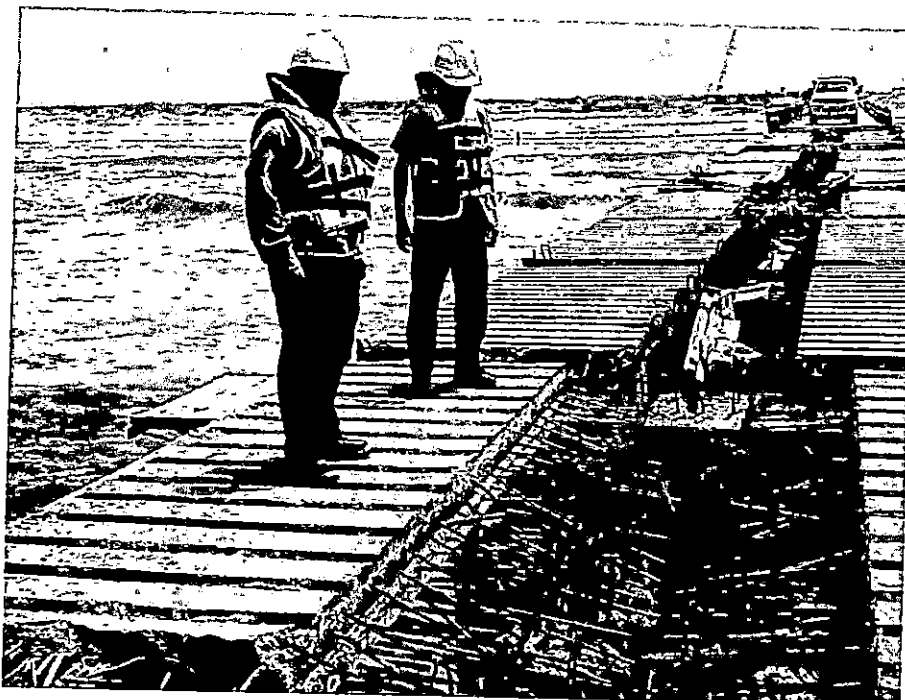
SUPERVISOR Y RESIDENTE EN EJE 174 – 175, SE OBSERVA DESCABEZADO DE PILOTES DE REFORZAMIENTO
